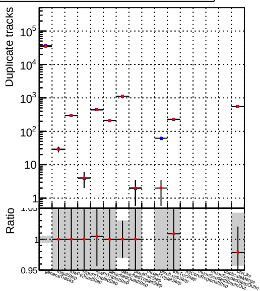
RECO Y 3 RECO
