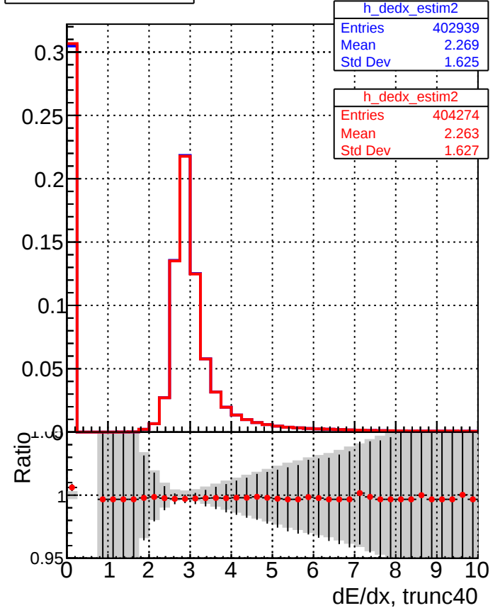
dE/dx estimator 2
