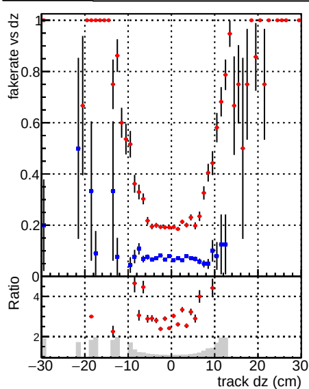
Global mkFitbase RECO DQM V0001_R000000001 Global CMSSW X Y Z DQM V0001_R000000001 Global CMSSW X Y Z
