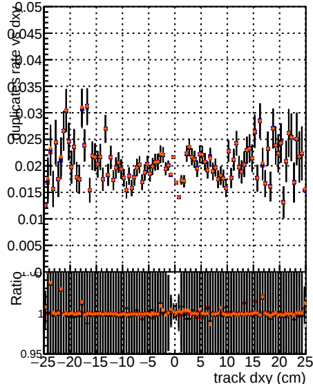
\text{mkFitNDOF}_2 - \text{RECO}
