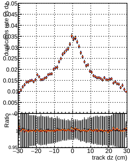
\text{mkFitNDOF}_2 - \text{RECO}
