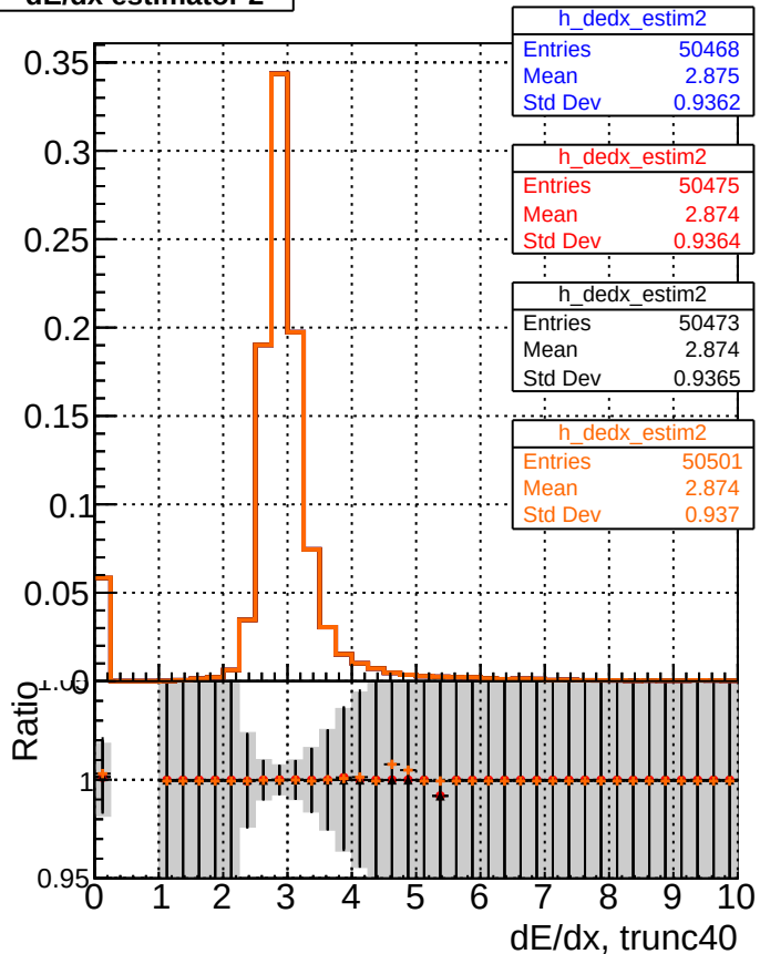
dE/dx estimator 2
