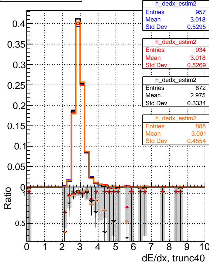
dE/dx estimator 2
