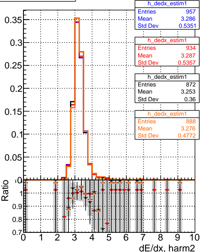
dE/dx estimator 1
