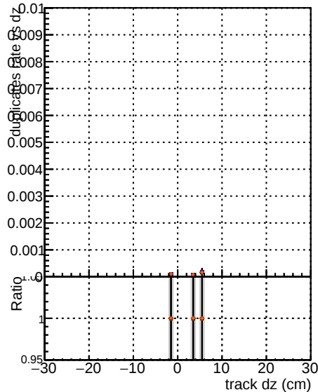
al=mkFitNBOF2-RECO
