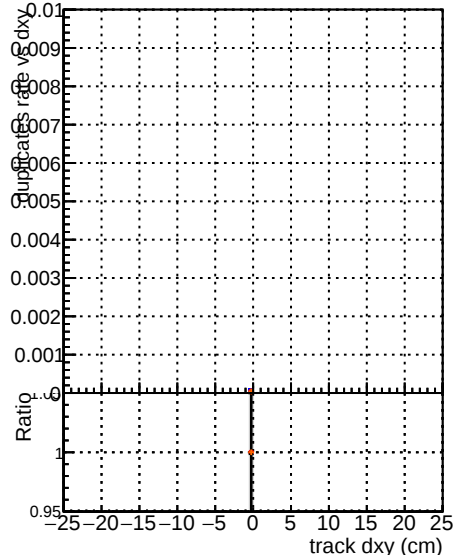
al=mkFitNBOF2-RECO
