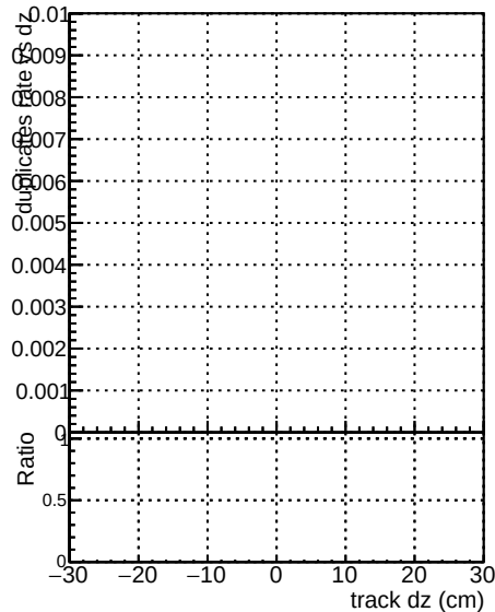
mkFitNBOF2 RECO
