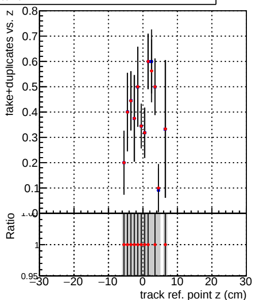
0timeHPTT
