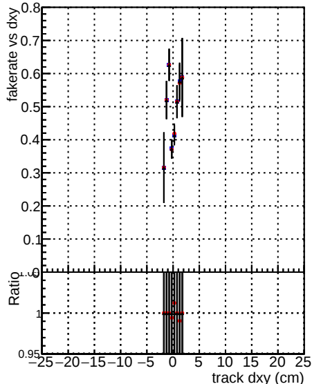
Fake rate vs d d HPTT PLAs CMSSW 0 0.35 0.25 0.15 1 0.30 0.22 0.12 2 0.25 0.18 0.10 3 0.20 0.15 0.08 4 0.18 0.13 0.07 5 0.15 0.11 0.06 6 0.13 0.09 0.05 7 0.11 0.08 0.04 8 0.10 0.07 0.03 9 0.09 0.06 0.02 10 0.08 0.05 0.02 DOM V0001 R0000000001 Global CMSSW 100ti DOM V0001 R0000000001 Global CMSSW 100timeHPTT DOM V0001 R0000000001 Global CMSSW 100timePLa
