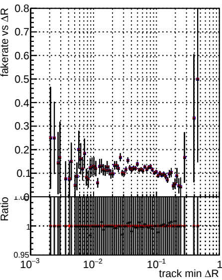
Legend: - DQM TT original - DQM TT originalCustomized - DQM TT noCutCustomized
