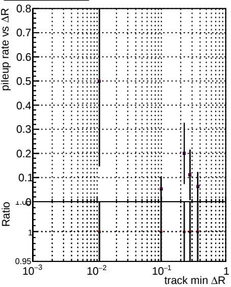
Legend: DQM TT original (black), DQM TT VLooseNEW (red), DQM TT VLooseNEW3iter (grey)
