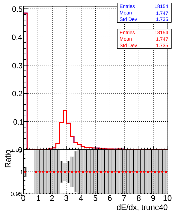
dE/dx estimator 2
