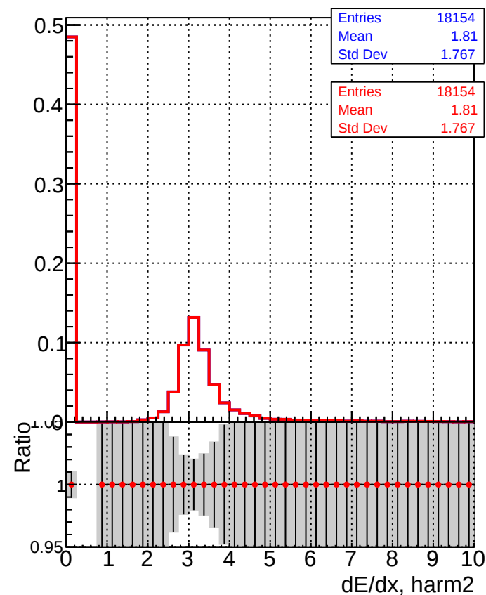
dE/dx estimator 1
