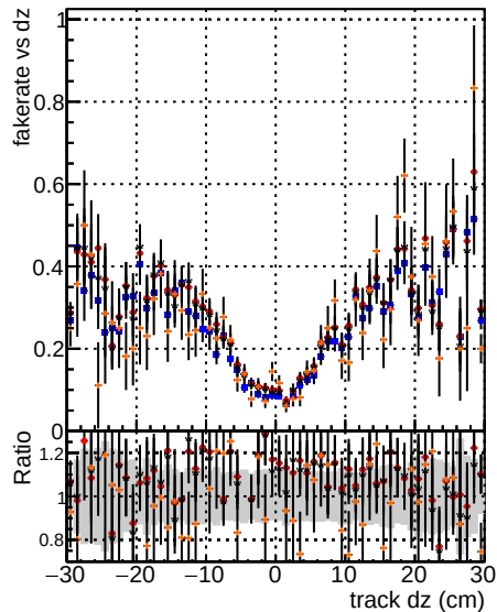
Fake rate vs dz DQM V0001 Global mxFit baseline DQM V0001 Global mxFit var DQM V0001 Global mxFit core30max DQM V0001 Global mxFit core30max+24DUPremoval
