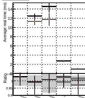
pixelLessStep
