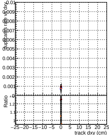
al=mkfilt|coreNoClean al=mkfilt|core50maxCa
