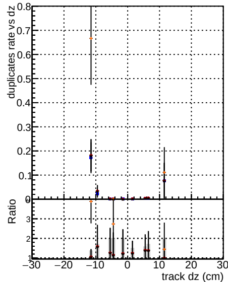
al=mkfilt|coreNoClean al=mkfilt|core50maxCa
