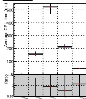
lowPtQuadStep
