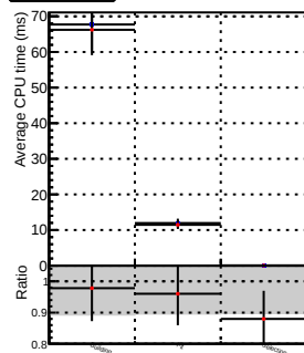
duplicateMerge
