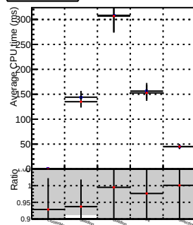
lowPtTripletStep
