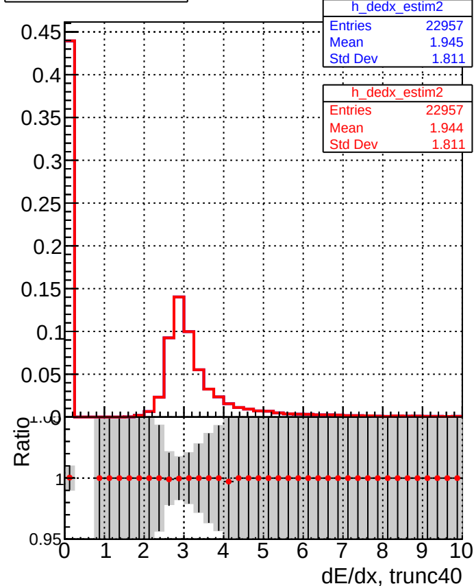
dE/dx estimator 2
