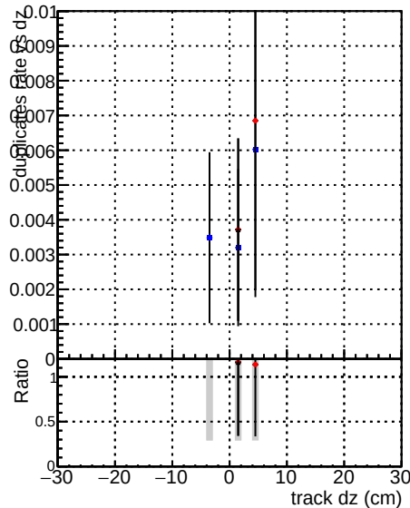
mkFit baseline al mkFit var al mkFit coreNoClean al mkFit coreSHits
