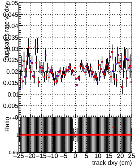
Global CMSSW_X_Y_Z all NODNN Global CMSSW_X_Y_Z all
