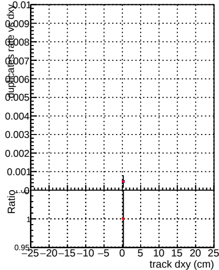
al CMSSW_X_Y_Z allNODNN al CMSSW_X_Y_Z all
