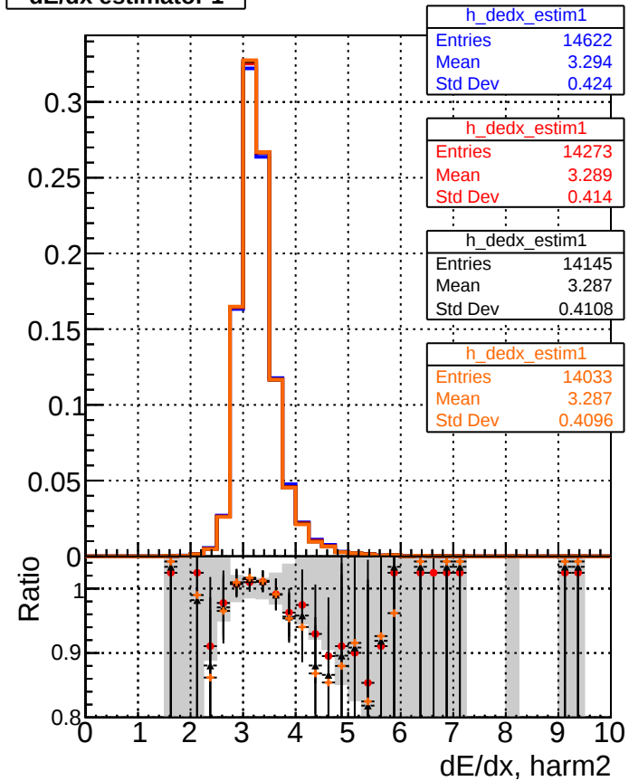
dE/dx estimator 1
