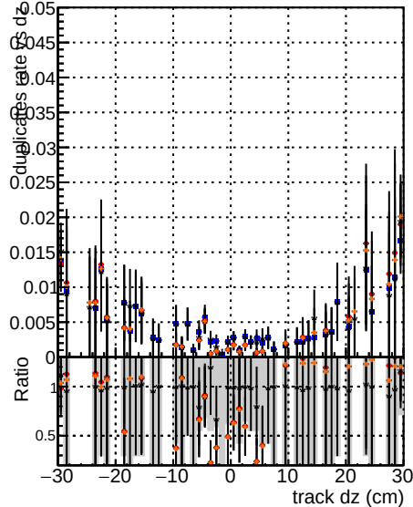
a|--mkfIt--mkswitch a|--mkfIt--CANDIkswitch
