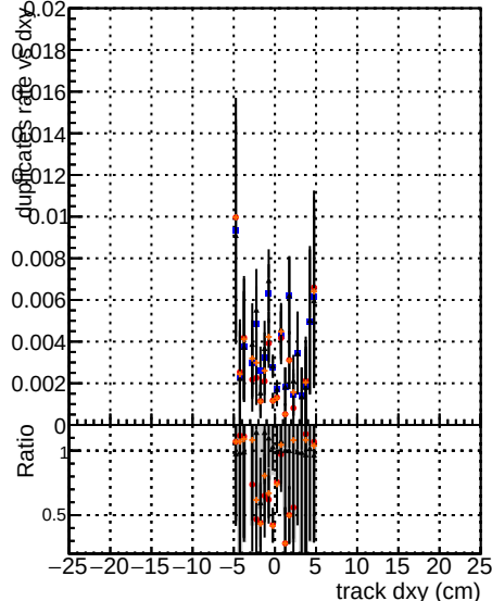
a|--mkfIt--mkswitch a|--mkfIt--CANDIkswitch
