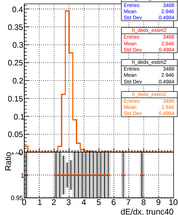
dE/dx estimator 2
