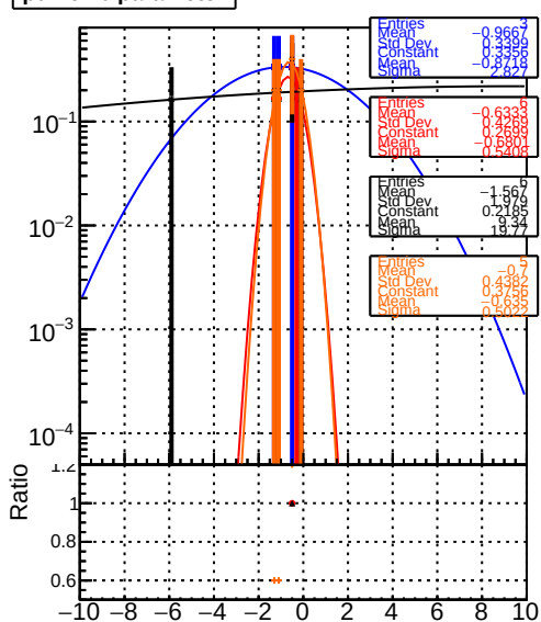
Rejection100 pull of \theta parameter
