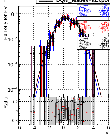
RecoPVAssoc
