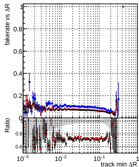
—●— DQM original —●— DQM testMkFitExport_initialStep —●— DQM testMkFitExportFit_initialStep
