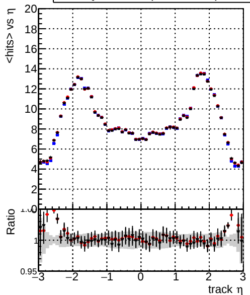
DQM_original DQM_testMkFitExport_initialStep DQM_testMkFitExportFit_initialStep mean hits
