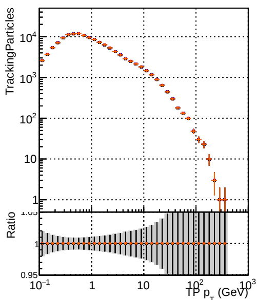
—●— DQM_original —●— DQM_original2 —●— DQM_testMkFitExport_initialStep —●— DQM_testMkFitExportFit_initialStep
