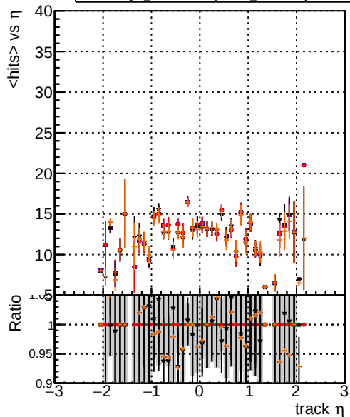
mean hit DQM_original DQM_original2 DQM_testMkFitExport_initialStep DQM_testMkFitExportFit_initialStep
