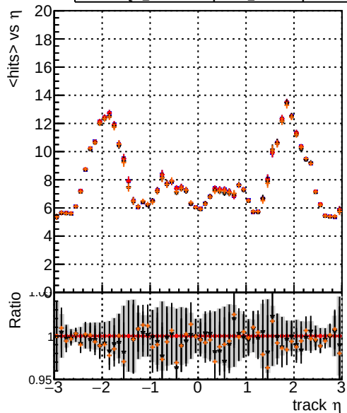
DQM_original DQM_original2 DQM_testMkFitExport_initialStep DQM_testMkFitExportFit_initialStep mean hit
