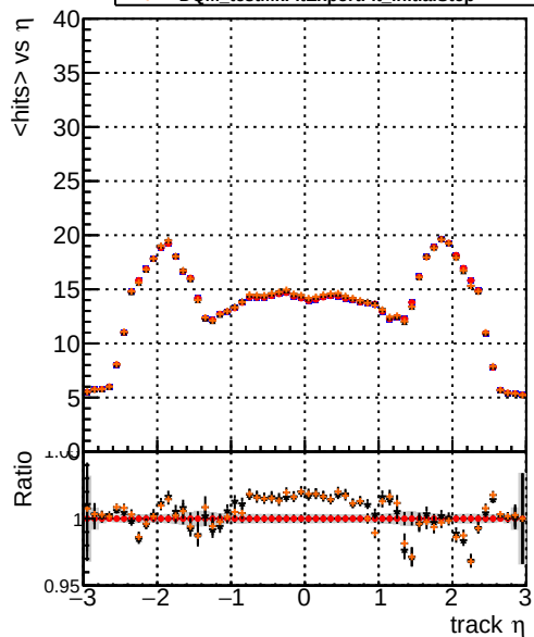
— DQM_original — DQM_original2 — DQM_testMkFitExport_initialStep — DQM_testMkFitExportFit_initialStep mean hits
