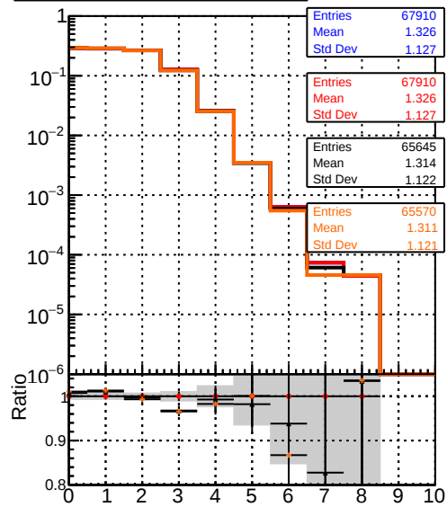
DQM_original DQM_original2 DQM_testMkFitExport_initialStep DQM_testMkFitExportFit_initialStep mean hits
