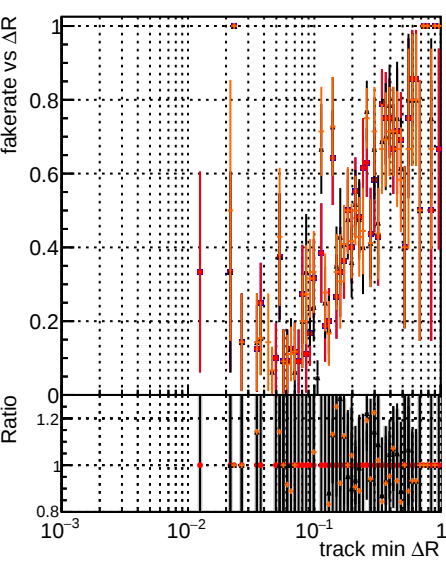
Fake rate vs \Delta R(\text{track, jet}) DQM original DQM original2 DQM testMKFitExport_initialStep DQM testMKFitExport_fit_initialStep
