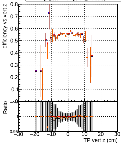
Efficiency vs vert z —●— DQM_original —●— DQM_original2 —●— DQM_testMkFitExport_initialStep —●— DQM_testMkFitExportFit_initialStep
