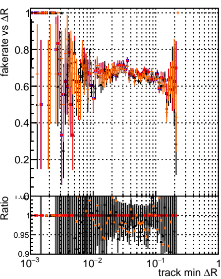
— DQM original — DQM original2 — DQM testMKFitExport_initialStep — DQM testMKFitExportFit_initialStep
