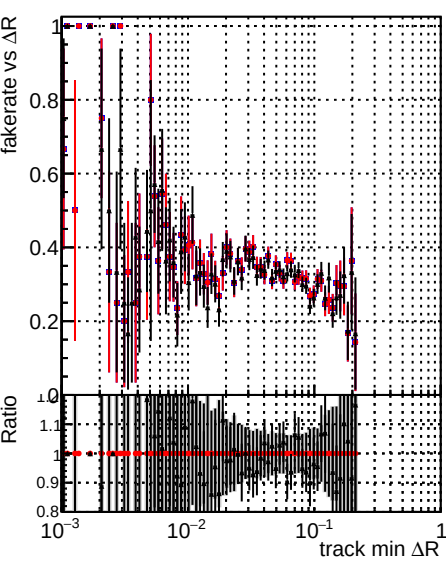
Legend: \blacksquare DQM original \bullet DQM original2 \blacktriangle DQM testMkFitExport_initialStep
