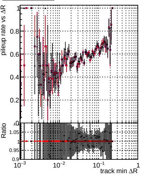
Legend: \blacksquare DQM original \bullet DQM original2 \blacktriangle DQM testMkFitExport_initialStep
