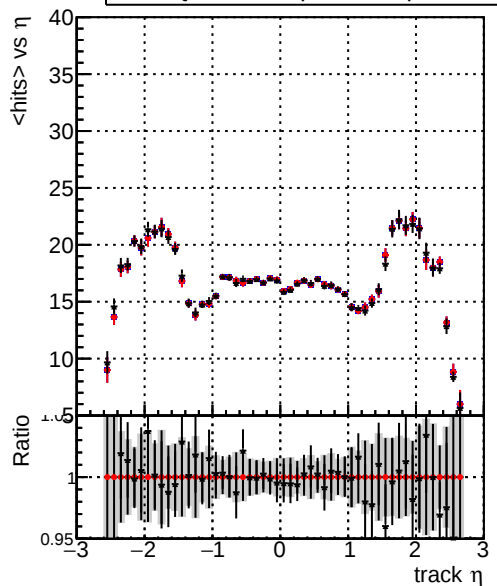
mean hits vs \eta — DQM_original — DQM_original2 — DQM_testMkFitExport_initialStep
