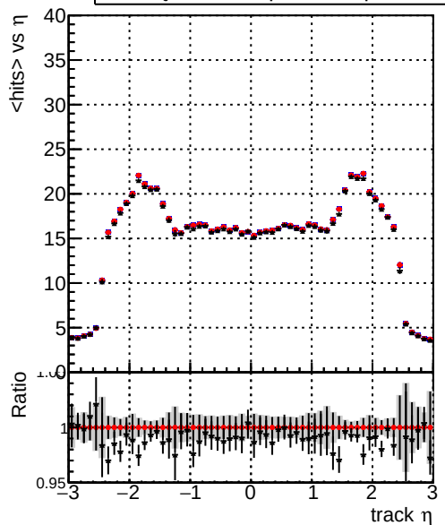
— DQM_original — DQM_original2 — DQM_testMkFitExport_initialStep mean hit
