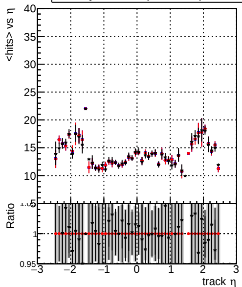
mean hits — DQM_original — DQM_original2 — DQM_testMkFitExport_initialStep
