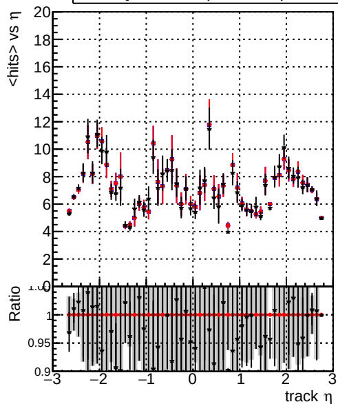
mean hit — DQM_original — DQM_original2 — DQM_testMkFitExport_initialStep
