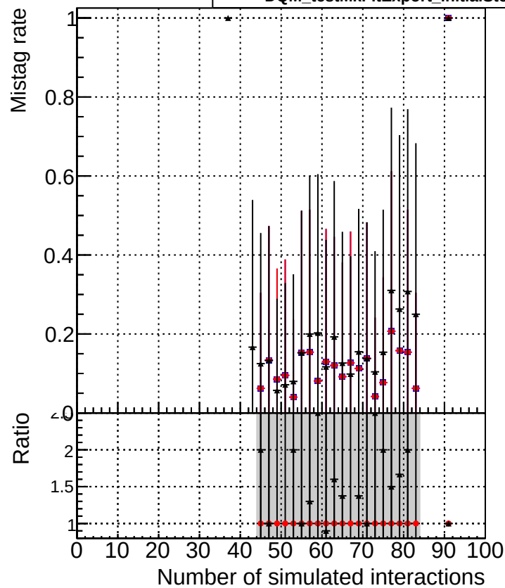
—•— DQM_original —•— DQM_original2 —•— DQM_testMkFitExport_initialStep
