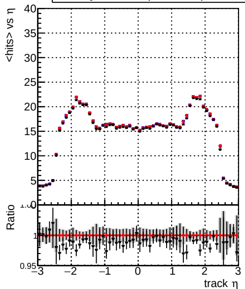
mean hit — DQM_original — DQM_original2 — DQM_testMkFitExport_initialStep
