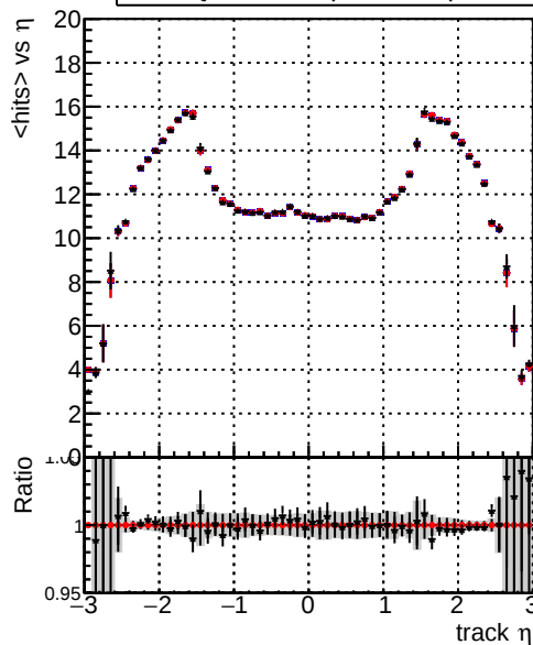
— DQM_original — DQM_original2 — DQM_testMkFitExport_initialStep mean hit
