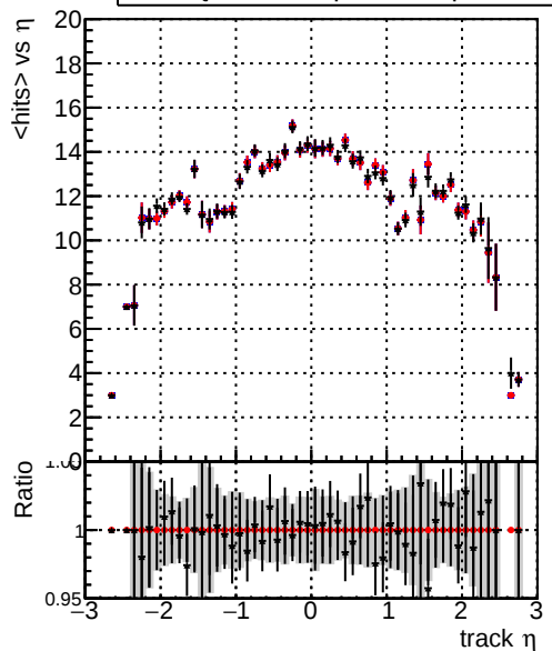
— DQM_original — DQM_original2 — DQM_testMkFitExport_initialStep mean hits
