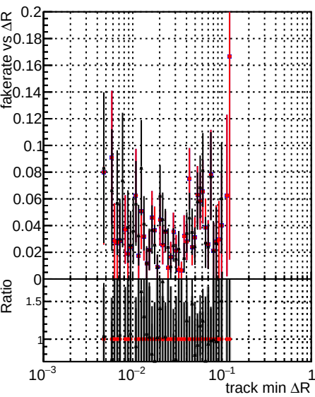
Fake rate vs \Delta R (track, jet) DQM original DQM original2 DQM testMkFitExport_initialStep
