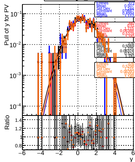
RecoPVAssoc2GenPVMatched_PullY
