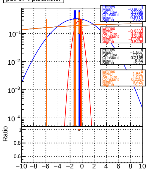
stSorting2 pull of \theta parameter
