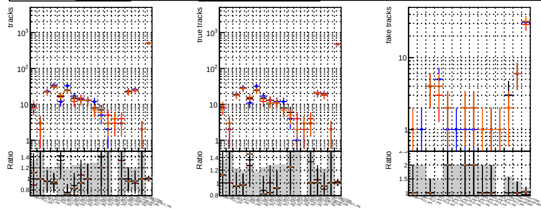
N of reco track vs. \chi^2 BQM original BQM testSorting1 BQM testSorting2 BQM testSorting3 BQM testSorting4 BQM testSorting5 BQM testSorting6 BQM testSorting7 BQM testSorting8 BQM testSorting9 BQM testSorting10 BQM testSorting11 BQM testSorting12 BQM testSorting13 BQM testSorting14 BQM testSorting15 BQM testSorting16 BQM testSorting17 BQM testSorting18 BQM testSorting19 BQM testSorting20 BQM testSorting21 BQM testSorting22 BQM testSorting23 BQM testSorting24 BQM testSorting25 BQM testSorting26 BQM testSorting27 BQM testSorting28 BQM testSorting29 BQM testSorting30 BQM testSorting31 BQM testSorting32 BQM testSorting33 BQM testSorting34 BQM testSorting35 BQM testSorting36 BQM testSorting37 BQM testSorting38 BQM testSorting39 BQM testSorting40 BQM testSorting41 BQM testSorting42 BQM testSorting43 BQM testSorting44 BQM testSorting45 BQM testSorting46 BQM testSorting47 BQM testSorting48 BQM testSorting49 BQM testSorting50 BQM testSorting51 BQM testSorting52 BQM testSorting53 BQM testSorting54 BQM testSorting55 BQM testSorting56 BQM testSorting57 BQM testSorting58 BQM testSorting59 BQM testSorting60 BQM testSorting61 BQM testSorting62 BQM testSorting63 BQM testSorting64 BQM testSorting65 BQM testSorting66 BQM testSorting67 BQM testSorting68 BQM testSorting69 BQM testSorting70 BQM testSorting71 BQM testSorting72 BQM testSorting73 BQM testSorting74 BQM testSorting75 BQM testSorting76 BQM testSorting77 BQM testSorting78 BQM testSorting79 BQM testSorting80 BQM testSorting81 BQM testSorting82 BQM testSorting83 BQM testSorting84 BQM testSorting85 BQM testSorting86 BQM testSorting87 BQM testSorting88 BQM testSorting89 BQM testSorting90 BQM testSorting91 BQM testSorting92 BQM testSorting93 BQM testSorting94 BQM testSorting95 BQM testSorting96 BQM testSorting97 BQM testSorting98 BQM testSorting99 BQM testSorting100
