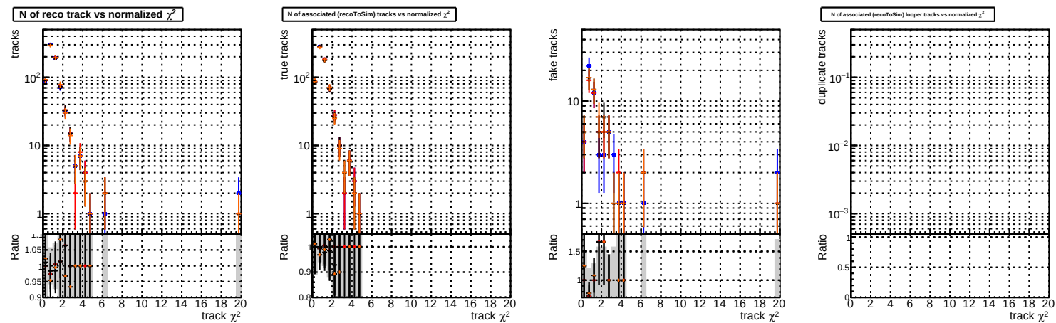
N of reco track vs. \chi^2 BQM original BQM testSorting1 BQM testSorting2 BQM testSorting3 BQM testSorting4 BQM testSorting5 BQM testSorting6 BQM testSorting7 BQM testSorting8 BQM testSorting9 BQM testSorting10 BQM testSorting11 BQM testSorting12 BQM testSorting13 BQM testSorting14 BQM testSorting15 BQM testSorting16 BQM testSorting17 BQM testSorting18 BQM testSorting19 BQM testSorting20 BQM testSorting21 BQM testSorting22 BQM testSorting23 BQM testSorting24 BQM testSorting25 BQM testSorting26 BQM testSorting27 BQM testSorting28 BQM testSorting29 BQM testSorting30 BQM testSorting31 BQM testSorting32 BQM testSorting33 BQM testSorting34 BQM testSorting35 BQM testSorting36 BQM testSorting37 BQM testSorting38 BQM testSorting39 BQM testSorting40 BQM testSorting41 BQM testSorting42 BQM testSorting43 BQM testSorting44 BQM testSorting45 BQM testSorting46 BQM testSorting47 BQM testSorting48 BQM testSorting49 BQM testSorting50 BQM testSorting51 BQM testSorting52 BQM testSorting53 BQM testSorting54 BQM testSorting55 BQM testSorting56 BQM testSorting57 BQM testSorting58 BQM testSorting59 BQM testSorting60 BQM testSorting61 BQM testSorting62 BQM testSorting63 BQM testSorting64 BQM testSorting65 BQM testSorting66 BQM testSorting67 BQM testSorting68 BQM testSorting69 BQM testSorting70 BQM testSorting71 BQM testSorting72 BQM testSorting73 BQM testSorting74 BQM testSorting75 BQM testSorting76 BQM testSorting77 BQM testSorting78 BQM testSorting79 BQM testSorting80 BQM testSorting81 BQM testSorting82 BQM testSorting83 BQM testSorting84 BQM testSorting85 BQM testSorting86 BQM testSorting87 BQM testSorting88 BQM testSorting89 BQM testSorting90 BQM testSorting91 BQM testSorting92 BQM testSorting93 BQM testSorting94 BQM testSorting95 BQM testSorting96 BQM testSorting97 BQM testSorting98 BQM testSorting99 BQM testSorting100
