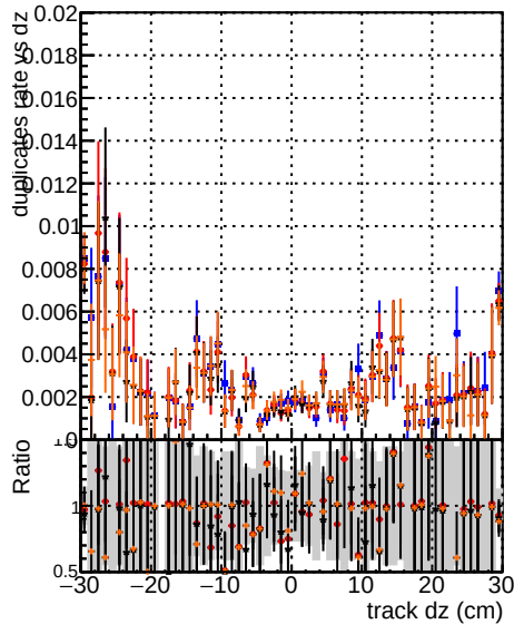
80 testSorting
